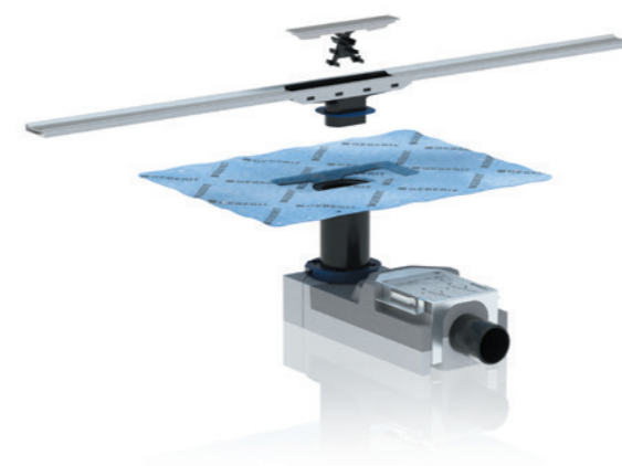
Souprava je k dispozici pro dvě výšky mazaniny: 90 – 220 mm s průtočnou kapacitou 0,8 l/s a 65 – 90 mm s průtočnou kapacitou 0,4 l/s.
